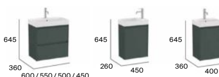
Unik compacto (lavabo y mueble)
