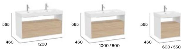
Mueble base para lavabo
